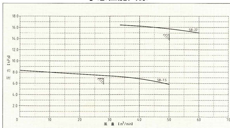
予想性能曲線
