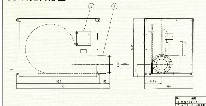
SB-7.5B外形図
