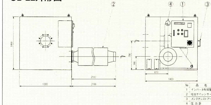
SB-22外形図
